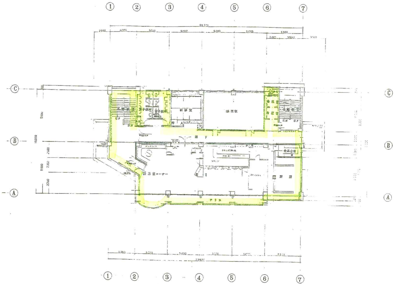
2階平面図 1/100
